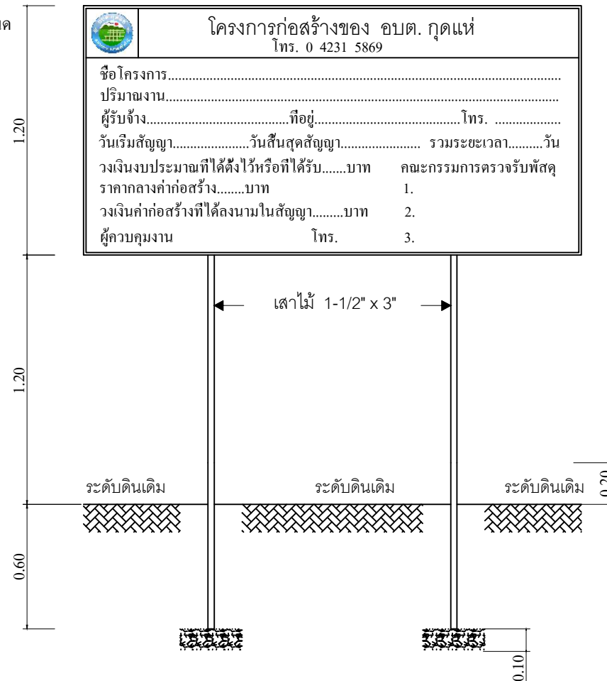
แบบป้ายโครงการระหว่างการก่อสร้าง 1: 25
