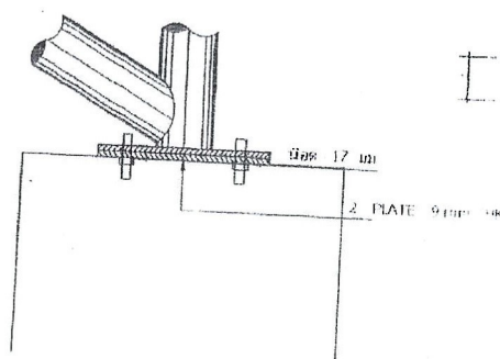
แบบที่ 2 (roller support) SCALE 1:10
