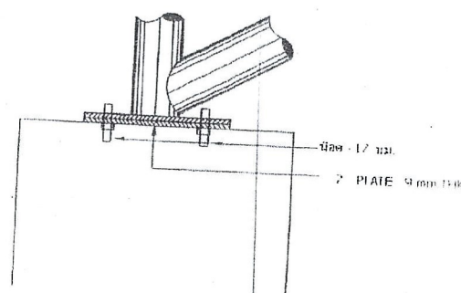
แบบที่ 1 (hinge support) SCALE 1:10
