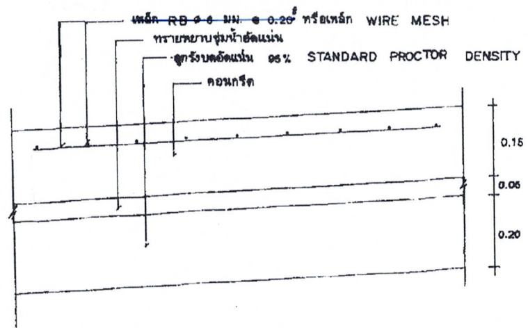
รายละเอียดคานคองกรีตเสริมเหล็ก NOT TO SCALE
