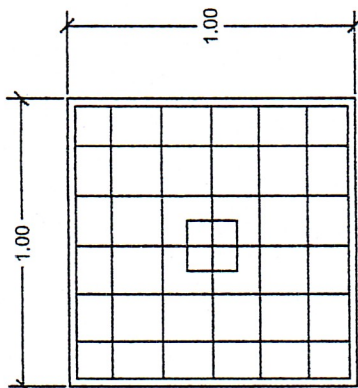
แปลนขยายฐานราก F1
